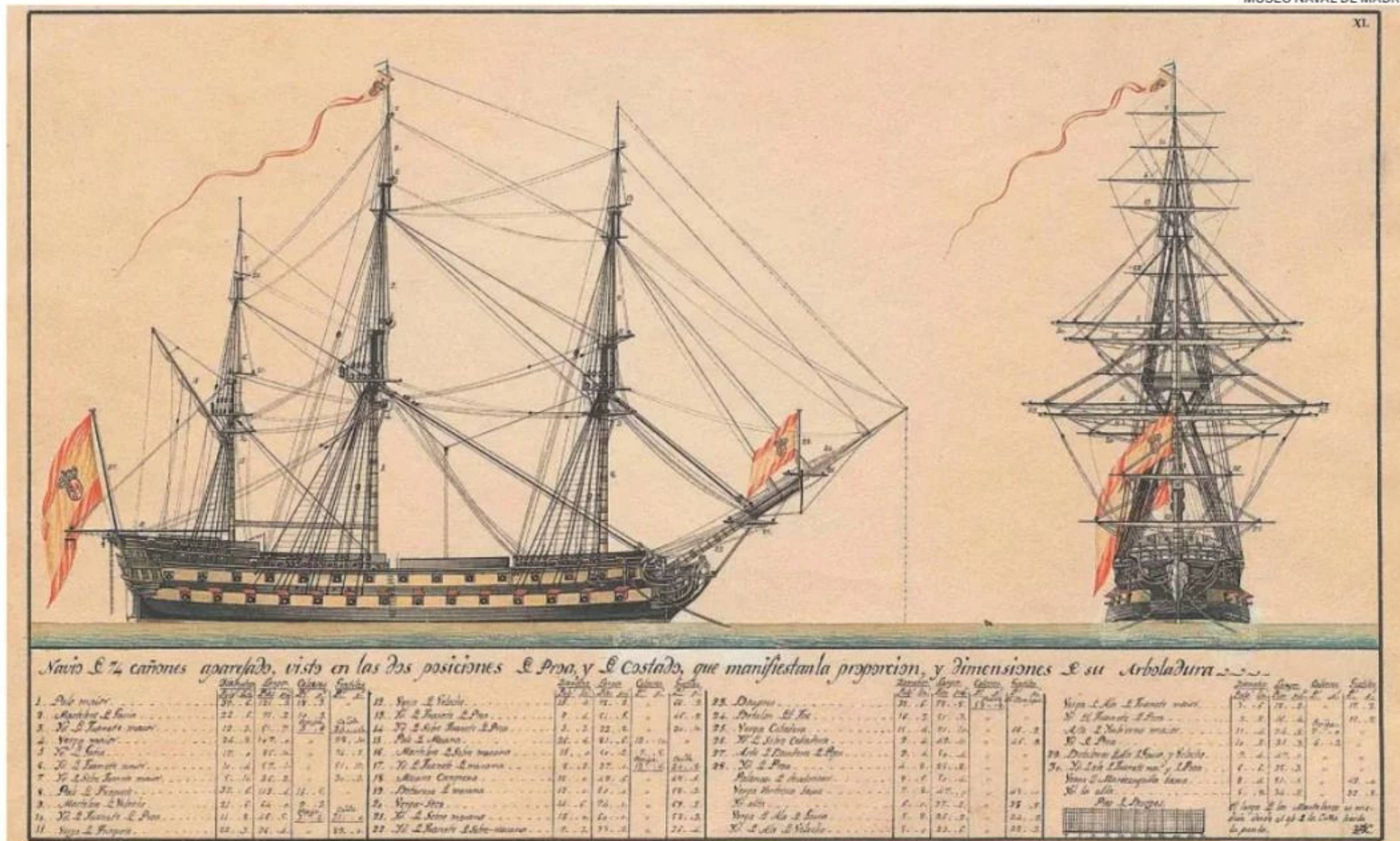
«Navío Montañés de 74 cañones aparejado» (1806), dibujo de Agustín Wauters y Horcasitas
